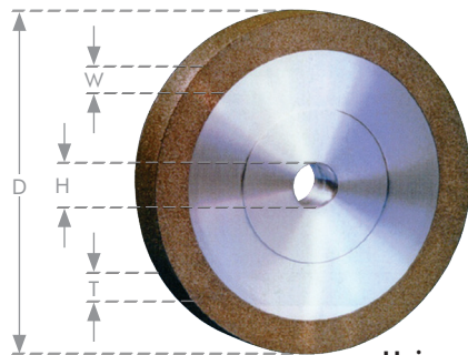
Universalschleifscheibe
